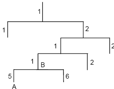
图 13-2 MIB 树结构
