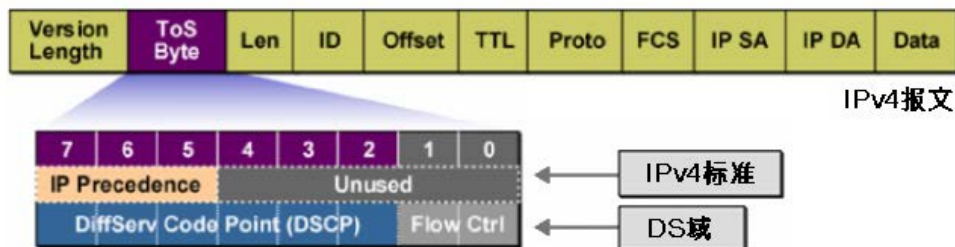
图 9-3 IP 报文
