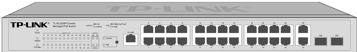
图 2-15 TL-SL3226P-Combo 的前面板
