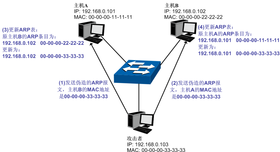
图 12-12 中间人攻击
