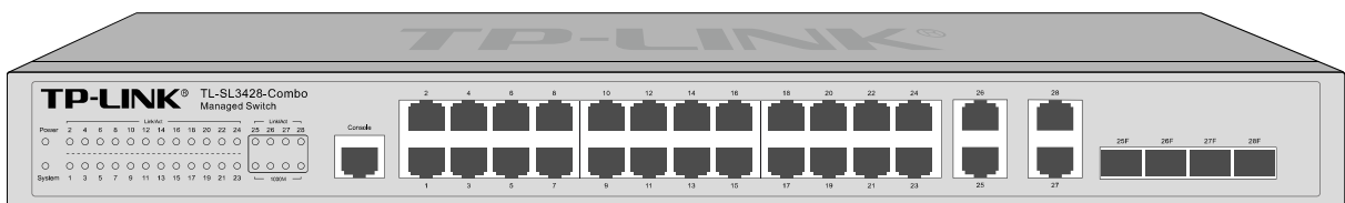
图 2-7 TL-SL3428-Combo 的前面板
