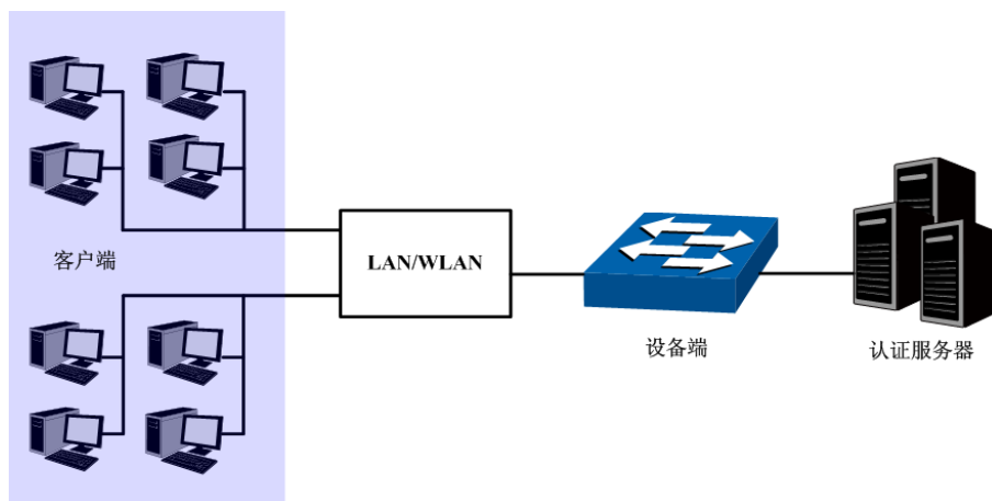
图 12-18 802.1X 认证的体系结构
