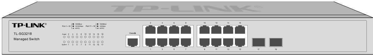
图 2-4 TL-SG3218 的前面板
