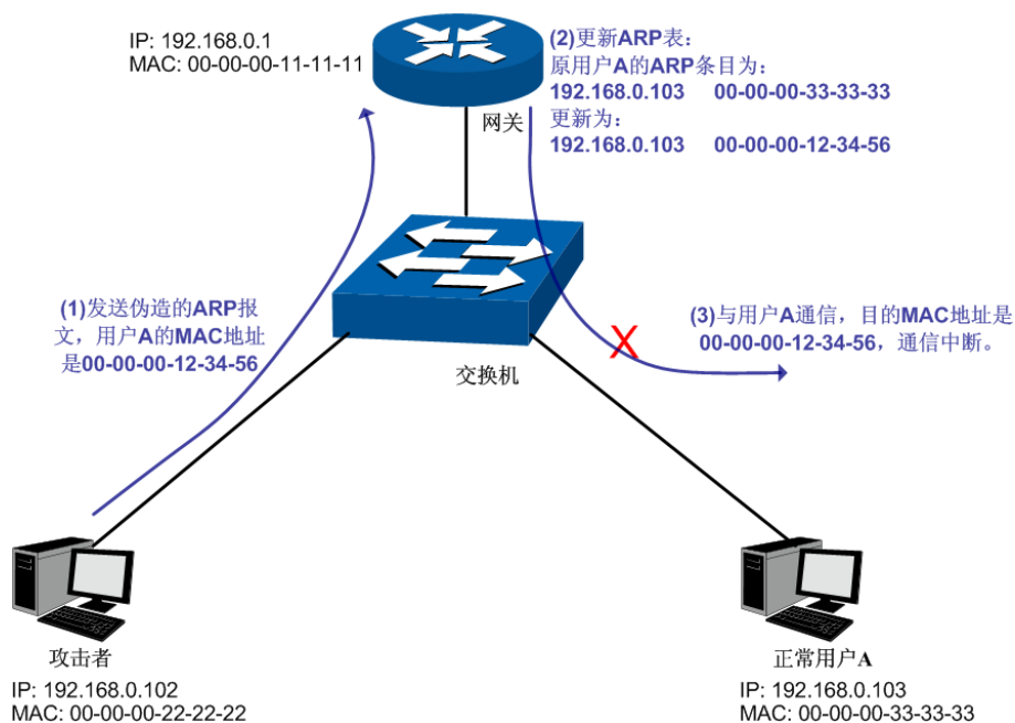
图 12-10 ARP 攻击-欺骗网关示意图
