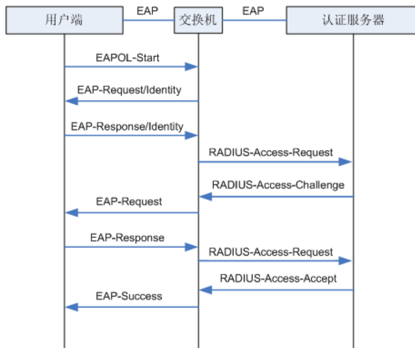
图 12-19 EAP-MD5 认证过程
