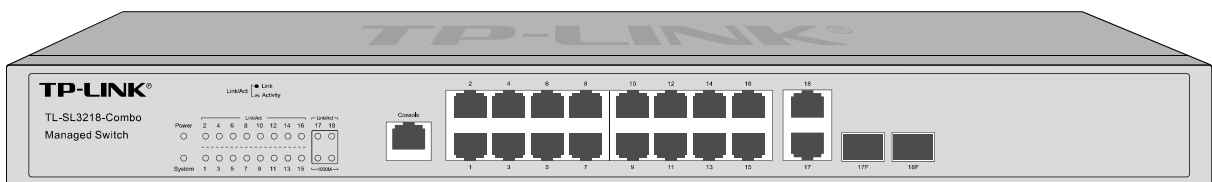
图 2-10 TL-SL3218-Combo 的前面板
