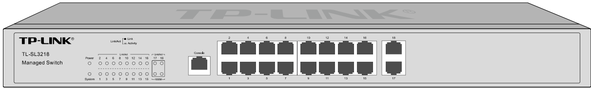
图 2-11 TL-SL3218 的前面板
