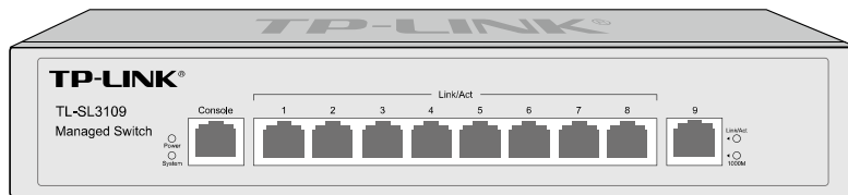
图 2-13 TL-SL3109 的前面板
