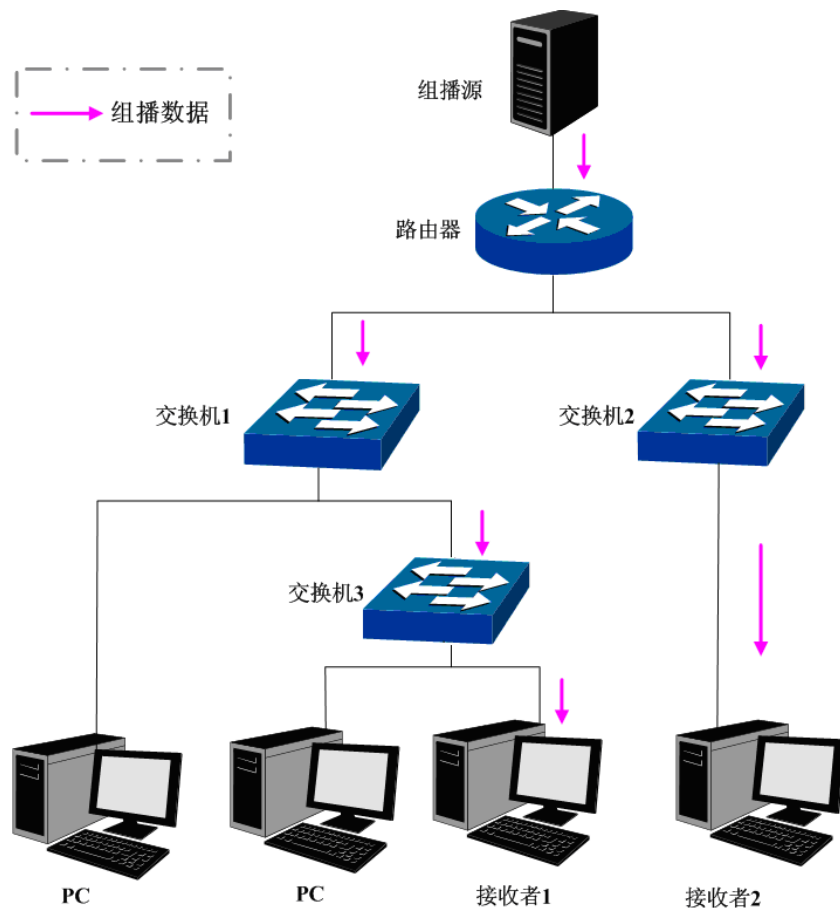
图 8-1 组播传输信息的方式
