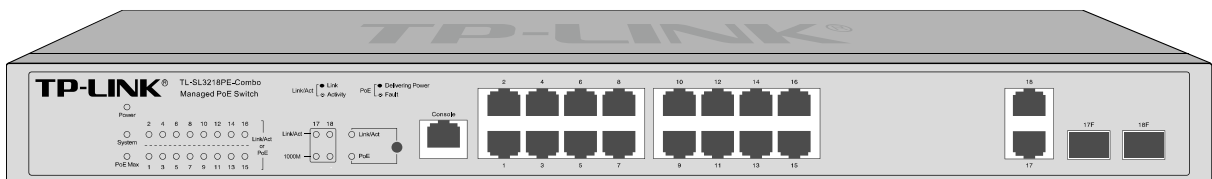
图 2-16 TL-SL3218PE-Combo 的前面板
