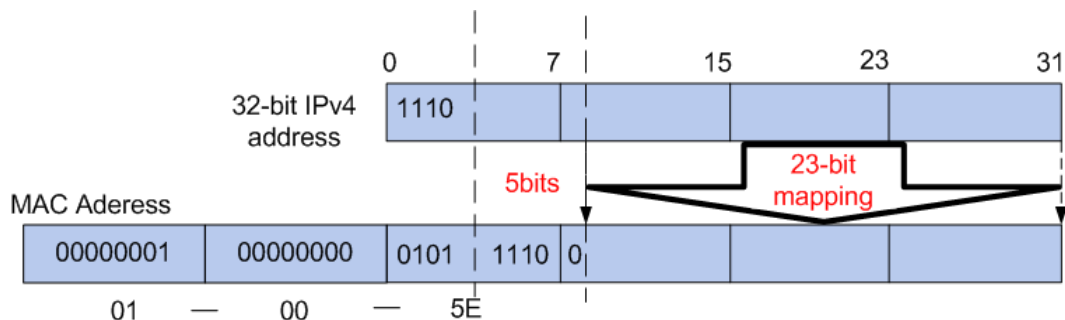
图 8-2 IPv4 组播 MAC 地址和组播 IP 地址的对应关系
